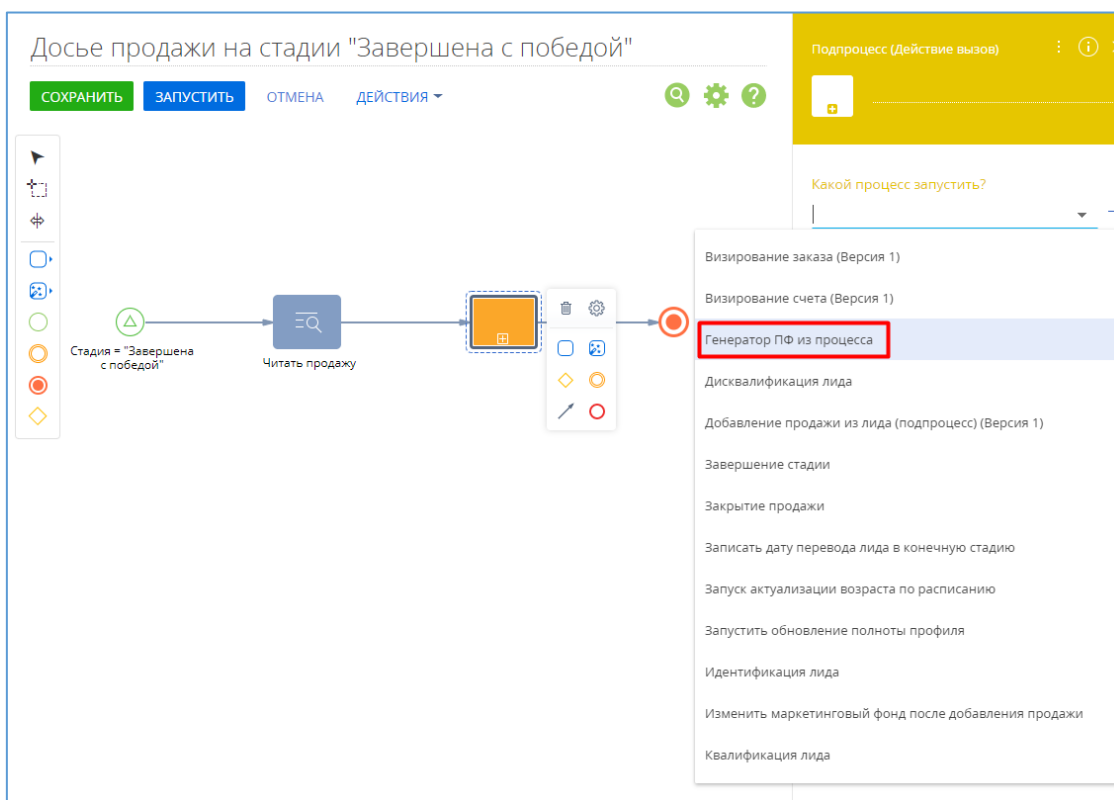
Рис. 2 – Настройка элемента «Подпроцесс (Действие вызов)»
